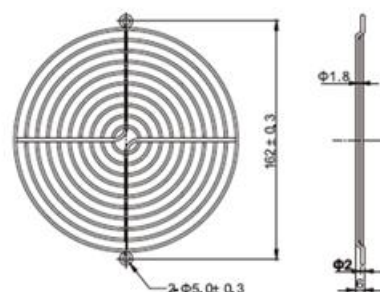
JL-15 For 150mm Fan
